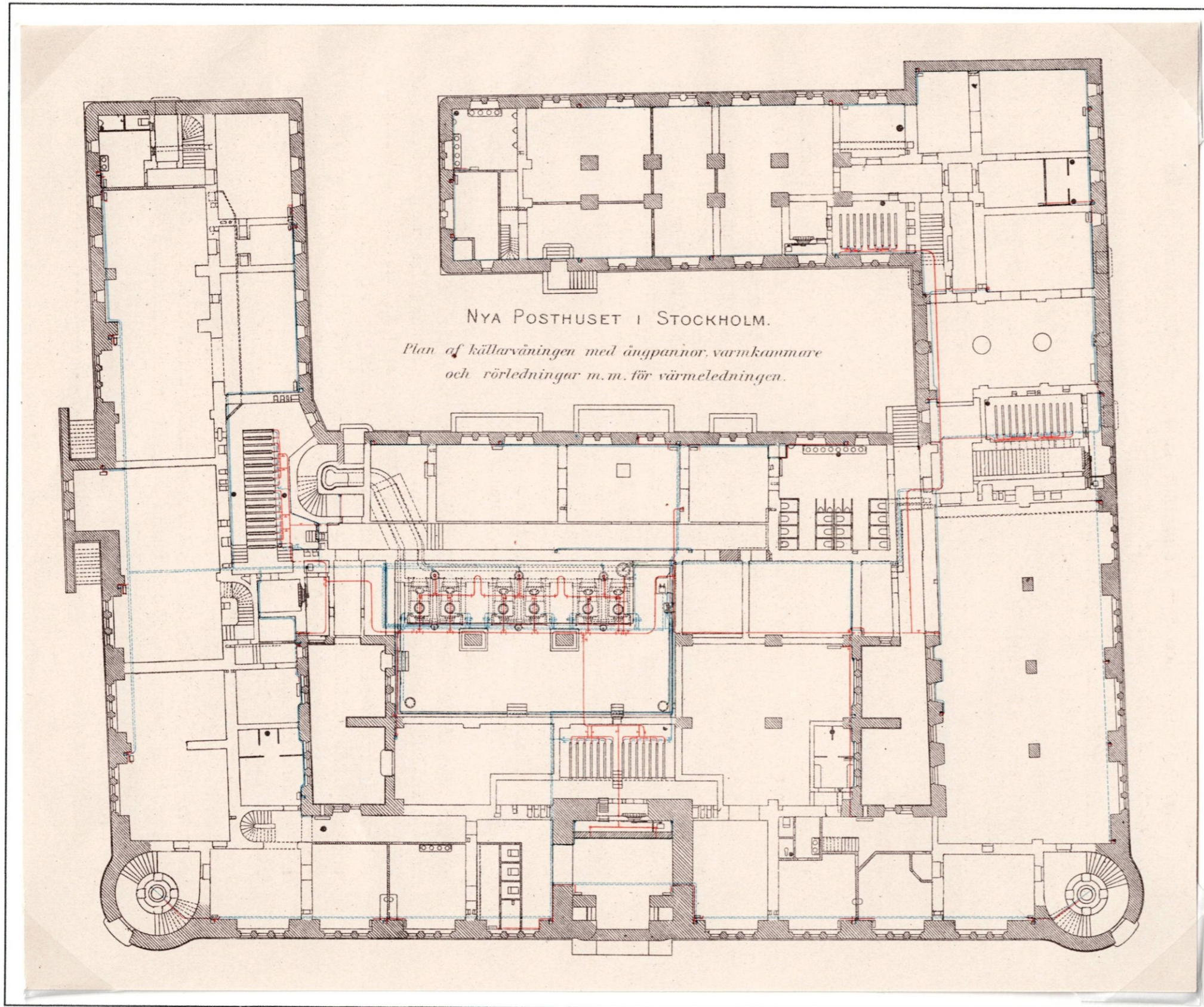
Ritning av källarvåningen med ångpannor varmkammare och värmeledningar
